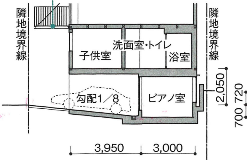
断面図[S=1:300]
